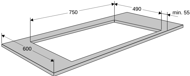
CARTESIO à encastrer
