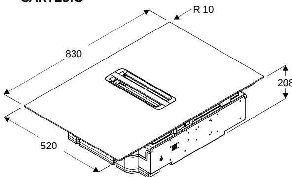
CARTESIO à fleur
