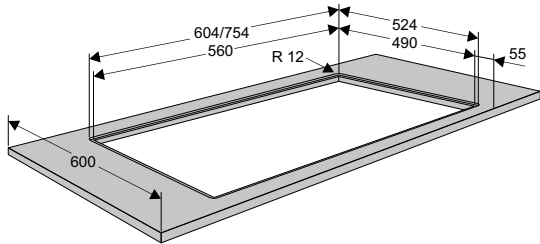
TOLOMEO 60 - 75 à fleur et à encastrer
