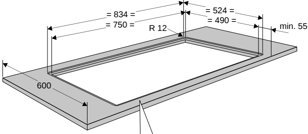
CARTESIO à encastrer
