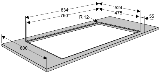
TOLOMEO 83 à fleur et à encastrer
