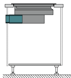
Installation sortie arrière
