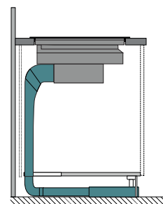
Installation sortie plinthe
